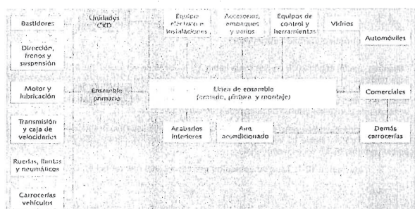
Ilustración 10-3: Proceso productivo del ensamble de vehículos
